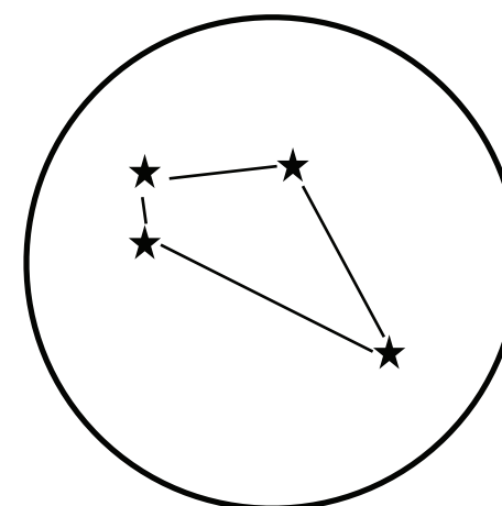
Sekstants
