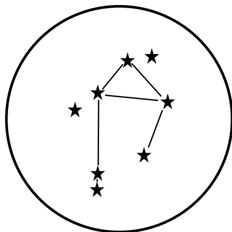
Svāri
