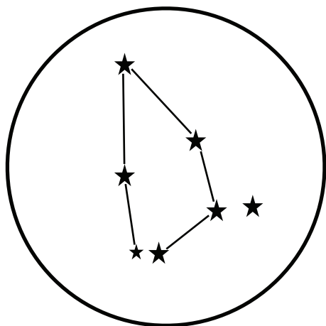
Cefejs
