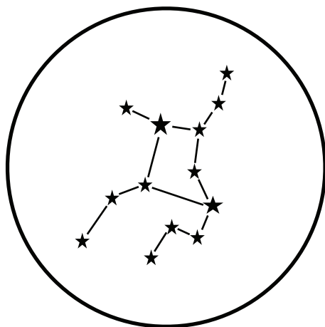
Jaunava
