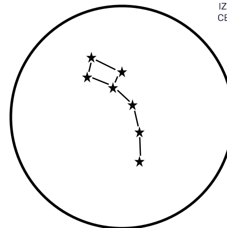
Mazais lācis
