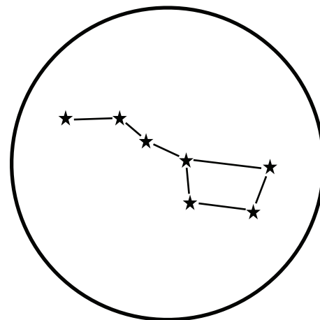
Lielais lācis
