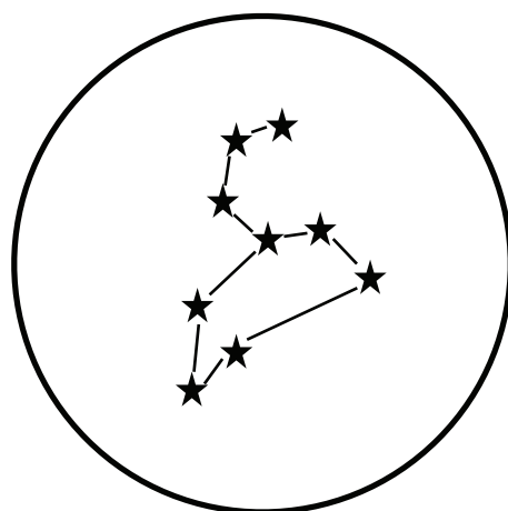
Lauva
